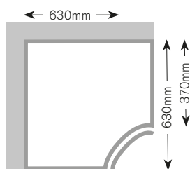
720mm High Door COCWU672
